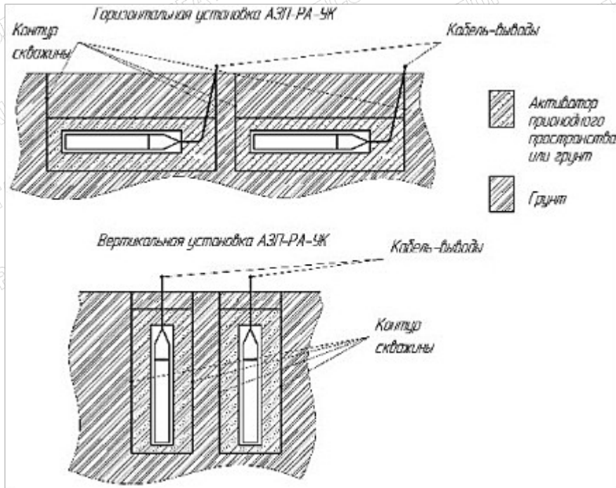
Установка АЗП-РА-УК
